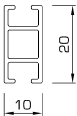
M92 - FOGA Mini - Upright or rail
