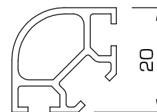
M92LR - FOGA Mini - Upright or rail, 90° corner
