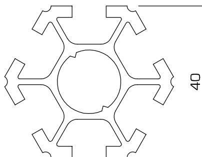
66 - Upright
