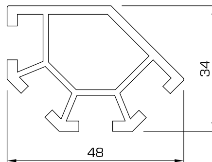
84 - Upright, 135°
