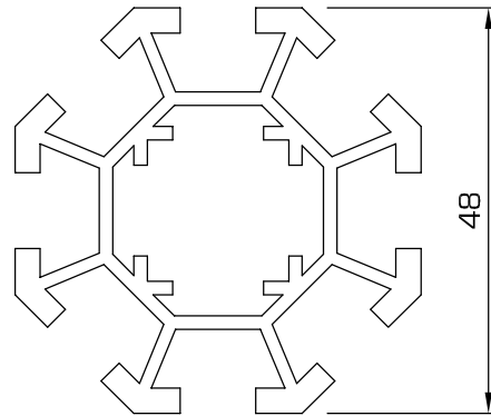
88 - Upright
