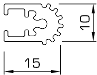
M21 - FOGA Mini - Gear edged, produces hinge
